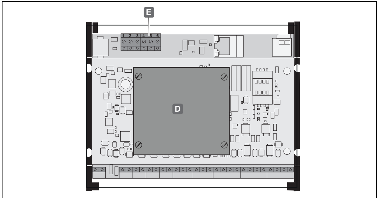
Fig. 10: Instalação do WTX 200 - ligado ao controlador
