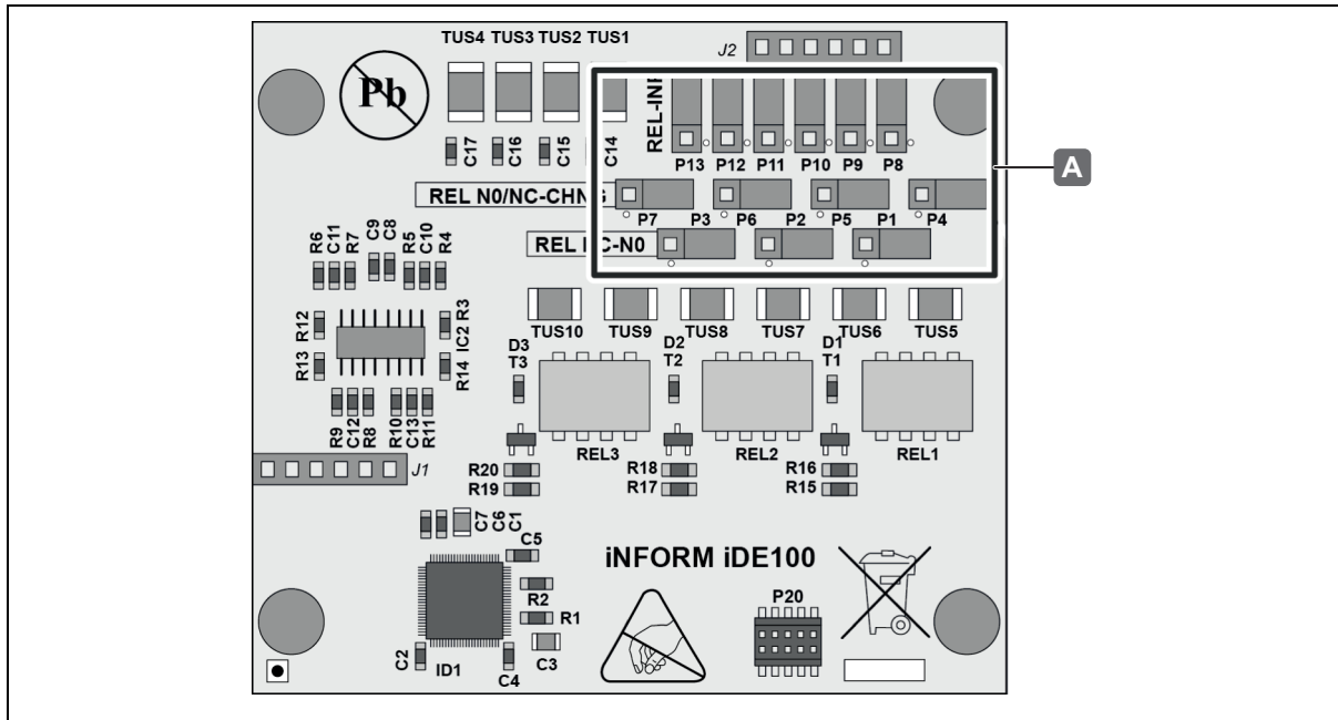
Fig. 18: WTX 200 - Posizione dei ponticelli in caso di utilizzo per altri ingressi analogici/digitali
