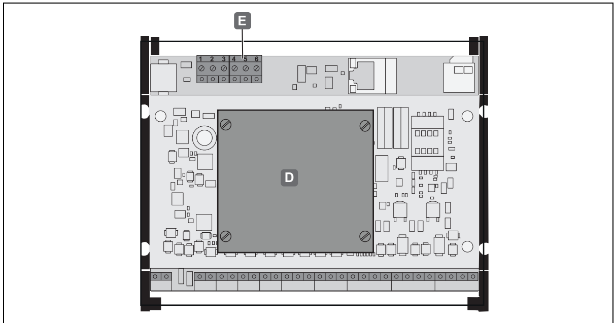
Fig. 10: Montaggio WTX 200 - inserito sul controller
