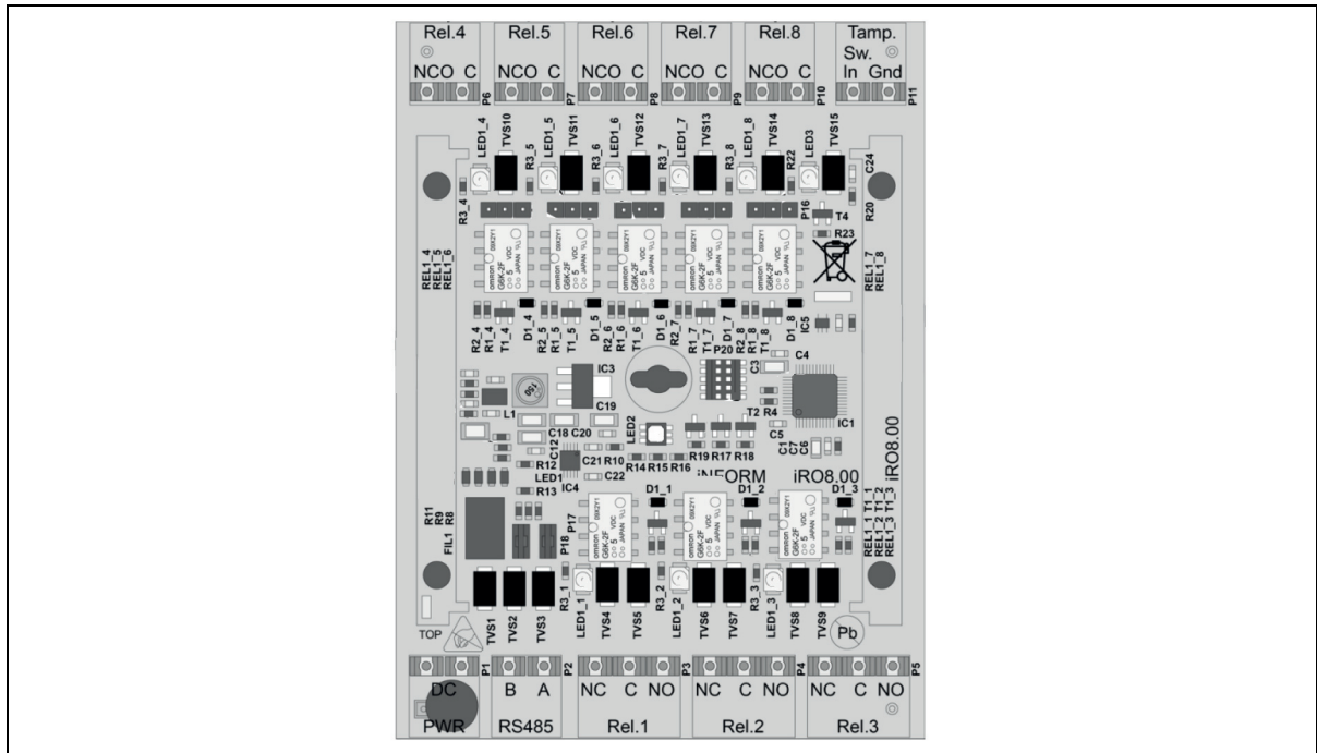
Ilustr. 4: WTX 201
