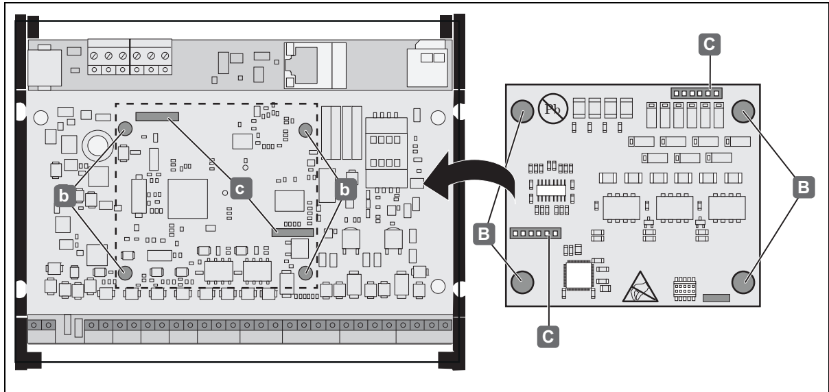
Ilustr. 9: Montaje WTX 200 - WTX 200 insertar en el controlador WTC 200
