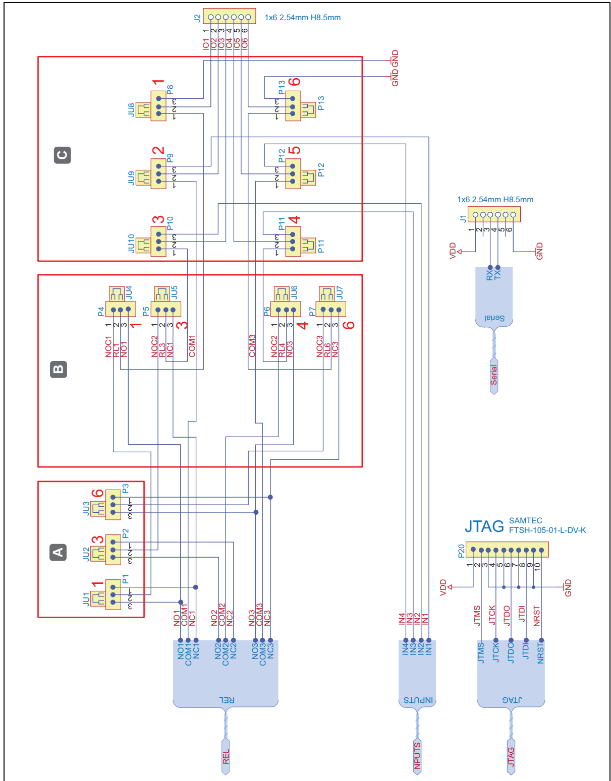
Fig. 16: Structure et affectation des broches de WTX 200
