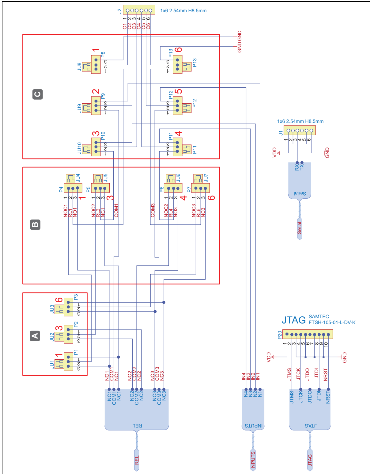
Fig. 16: Estrutura e atribuição de pinos do WTX 200
