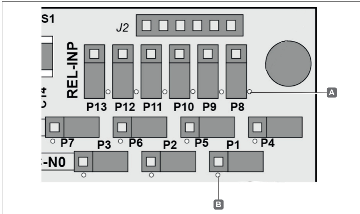
Fig. 17: Connessioni WTX 200- Posizione connessione n° 1 (punto bianco)
