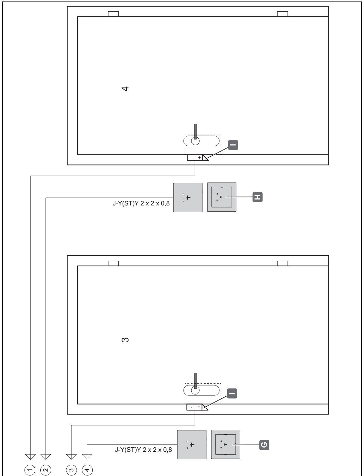
Ilustr. 32: Ejemplo de instalación 5 - Parte 2 - Cuatro puertas con un lector / abrepuertas y un controlador (incl. placa de ampliación)
