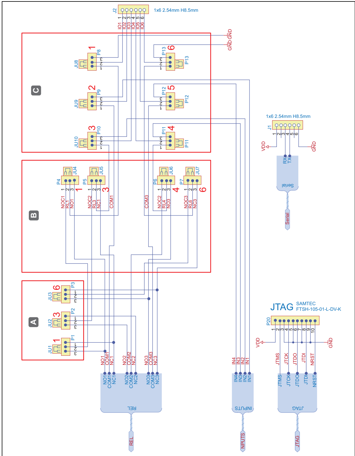
Fig. 16: Struttura e assegnazione pin del WTX 200
