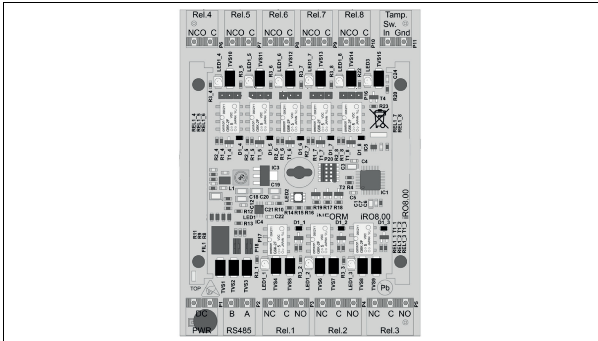
Abb. 4: WTX 201
