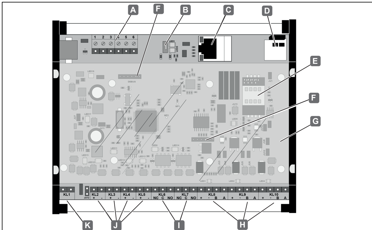
Fig. 14: Connessioni WTC 200
