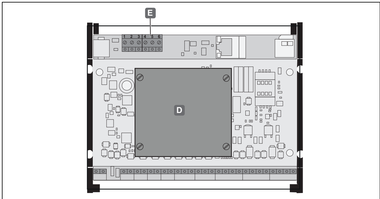
Abb. 10: Montage WTX 200 - auf Controller aufgesteckt
