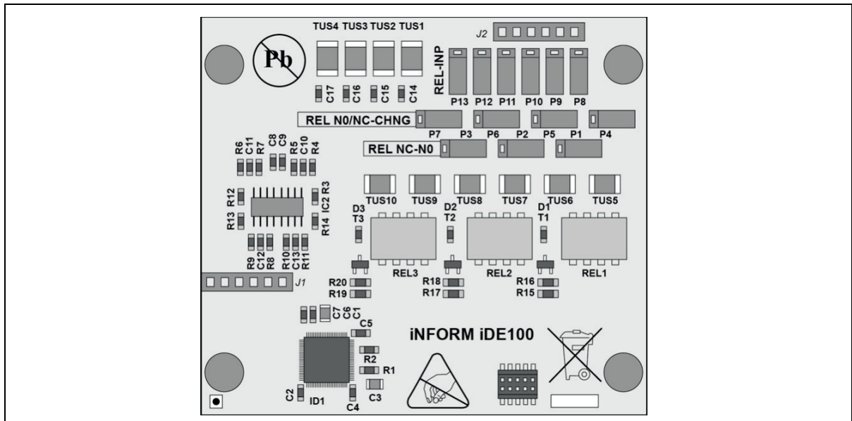
Fig. 2: WTX 200
