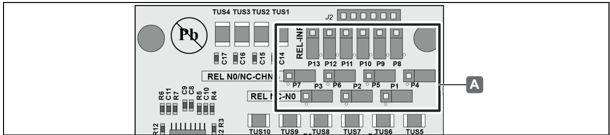
Fig. 7: Montaggio WTX 200 - Impostare il ponticello
