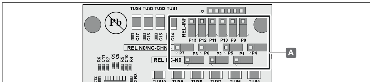
Fig. 7: Instalação do WTX 200 – configuração do conector
