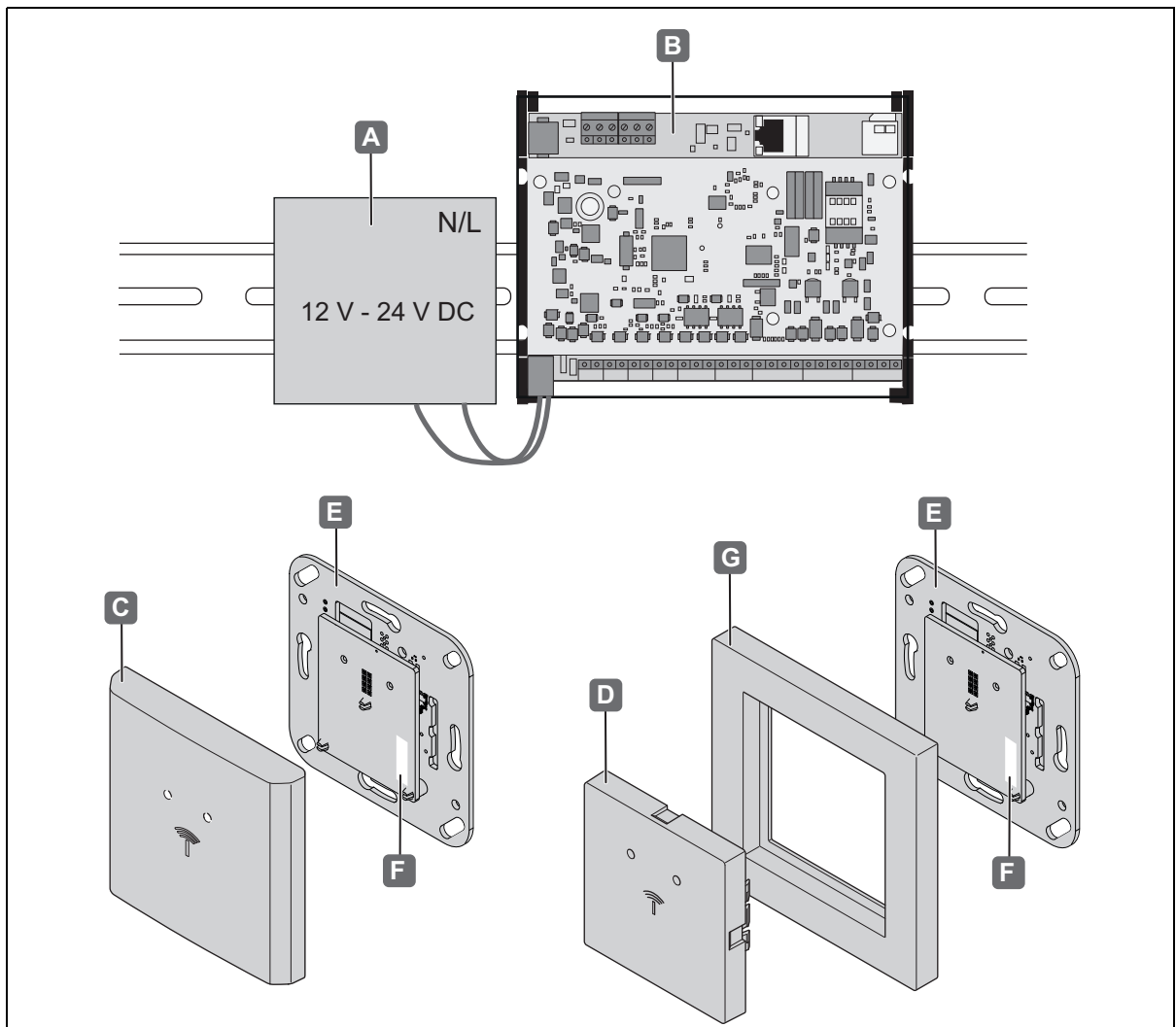
Abb. 1: Systemübersicht
