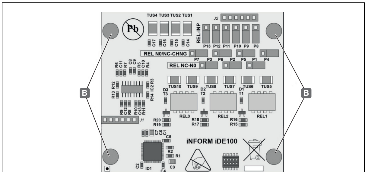
Fig. 8: Montaggio WTX 200 - applicare il distanziatore
