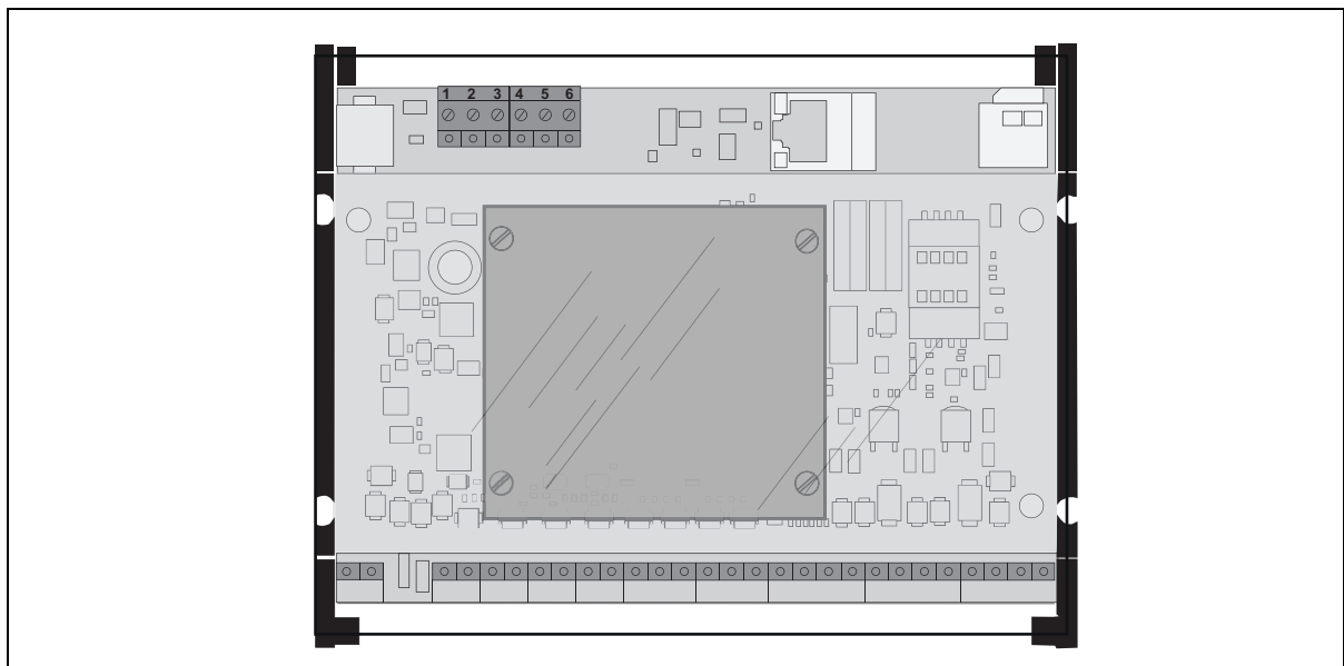
Fig. 3: WTX 200 - enfiché sur le contrôleur
