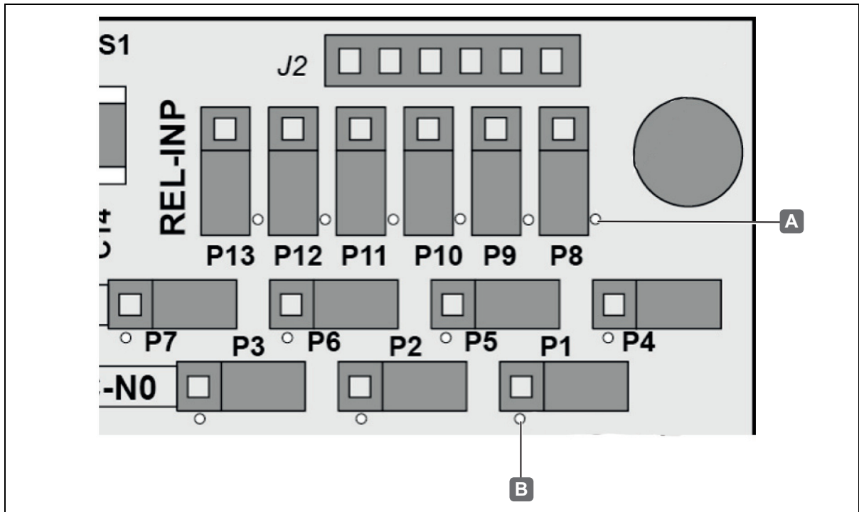
Abb. 17: Anschlüsse WTX 200- Position Anschluss Nr. 1 (weißer Punkt)
