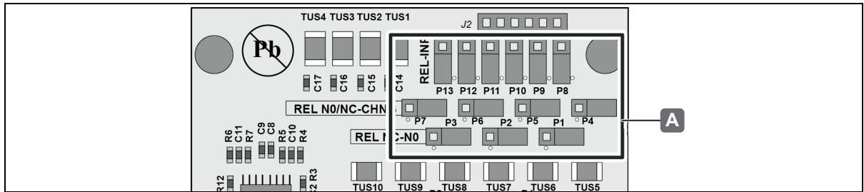
Abb. 7: Montage WTX 200 - Jumper setzen
