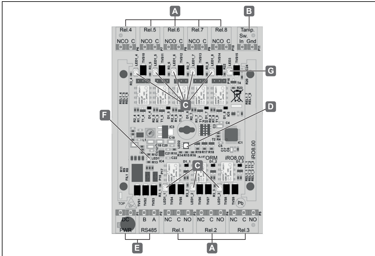
Fig. 20: Connessioni WTX 201
