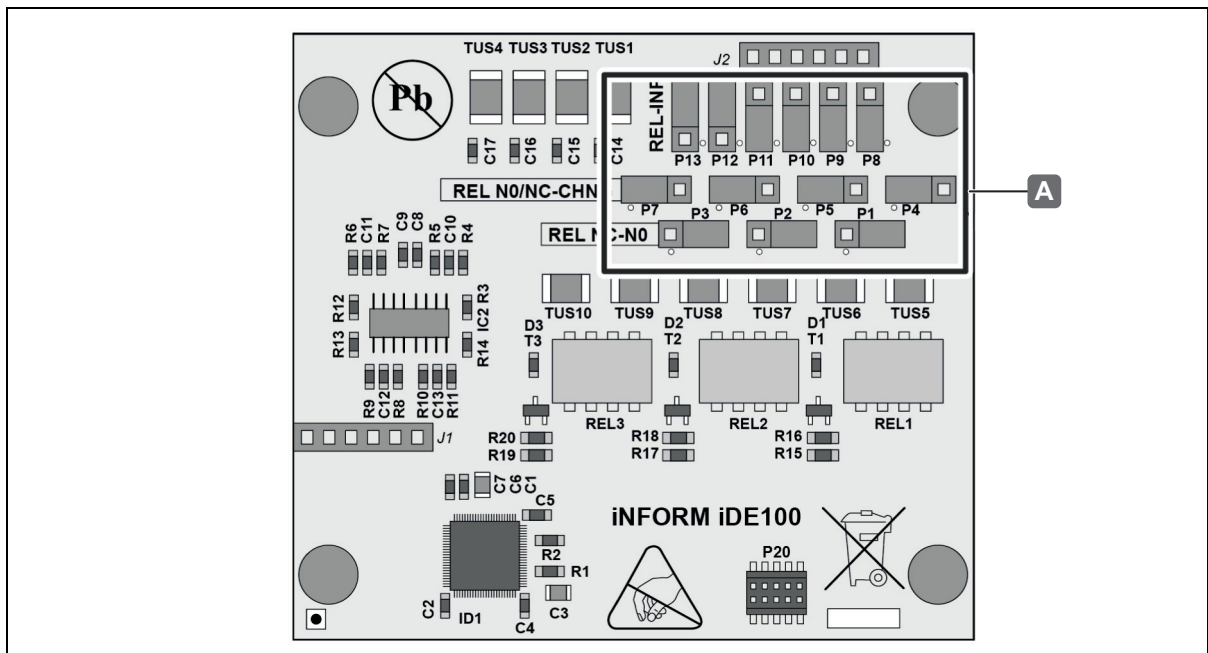
Abb. 19: WTX 200 – Position der Jumper bei Verwendung für 2 weitere Relaisausgänge und 1 weiteren Analog-/Digitaleingang
