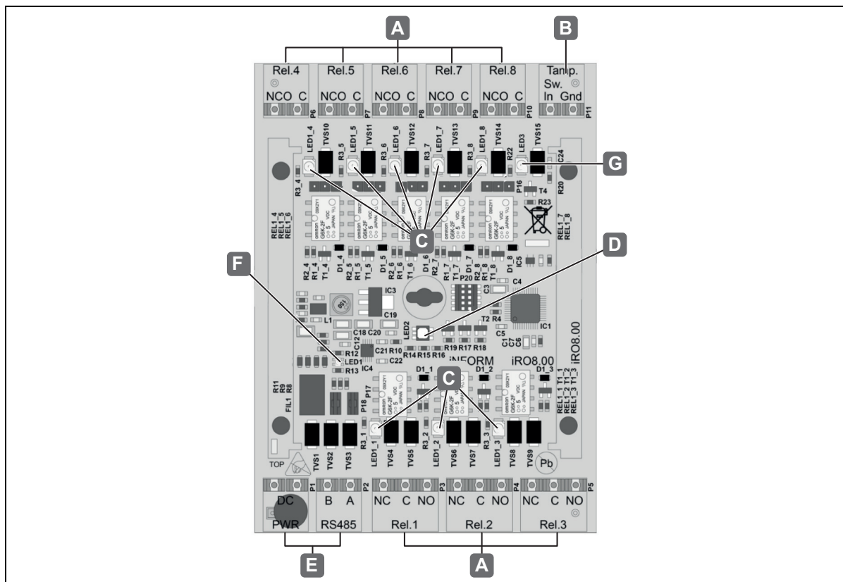
Ilustr. 20: Conexiones WTX 201
