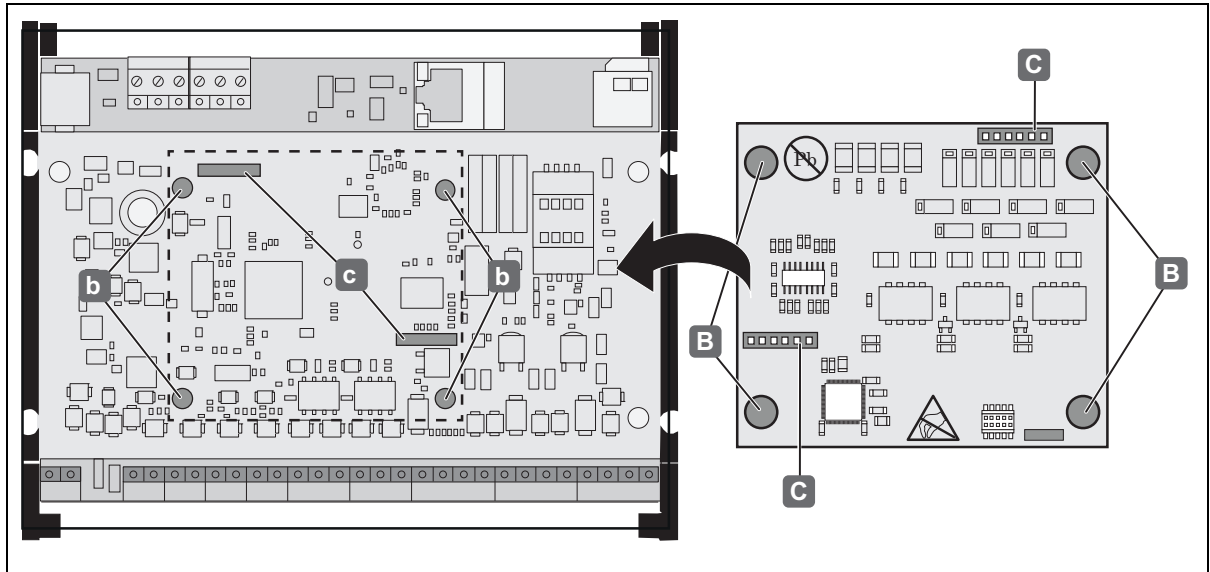
Fig. 9: Montage WTX 200 - WTX 200 Enficher WTC 200 sur le contrôleur
