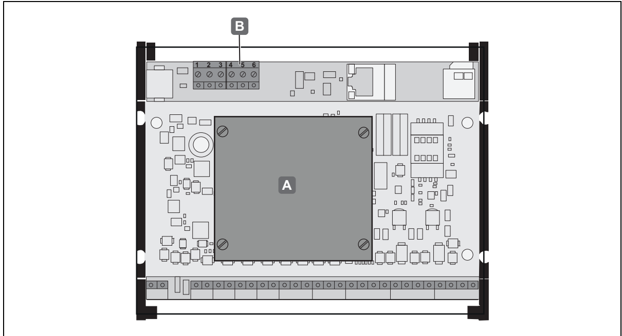
Ilustr. 15: Conexiones WTX 200
