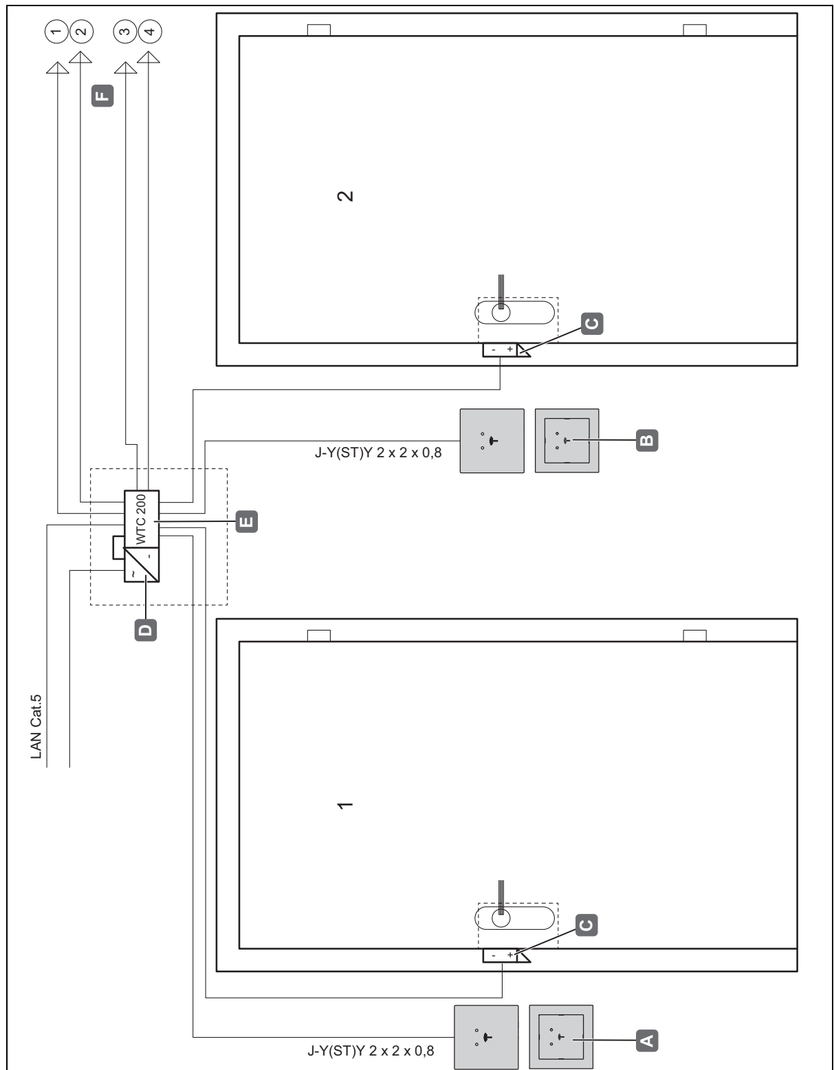
Fig. 31: Esempio di installazione 5 - Parte 1 - Quattro porte con ciascuna di un lettore / apriporta e un controller (incl. scheda di espansione)
