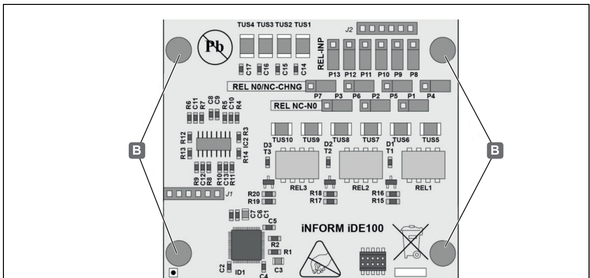
Abb. 8: Montage WTX 200 - Abstandshalter anbringen
