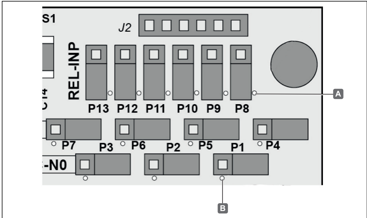
Fig. 17: Connexions WTX 200- Position connexion n°1 (point blanc)
