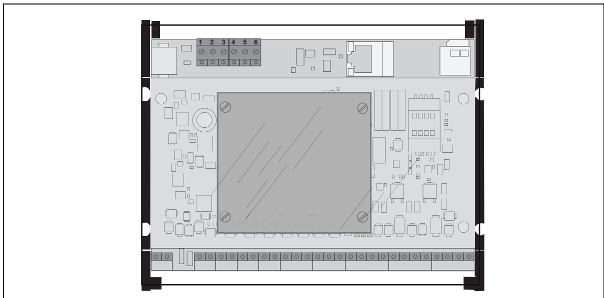
Abb. 3: WTX 200 - auf Controller aufgesteckt
