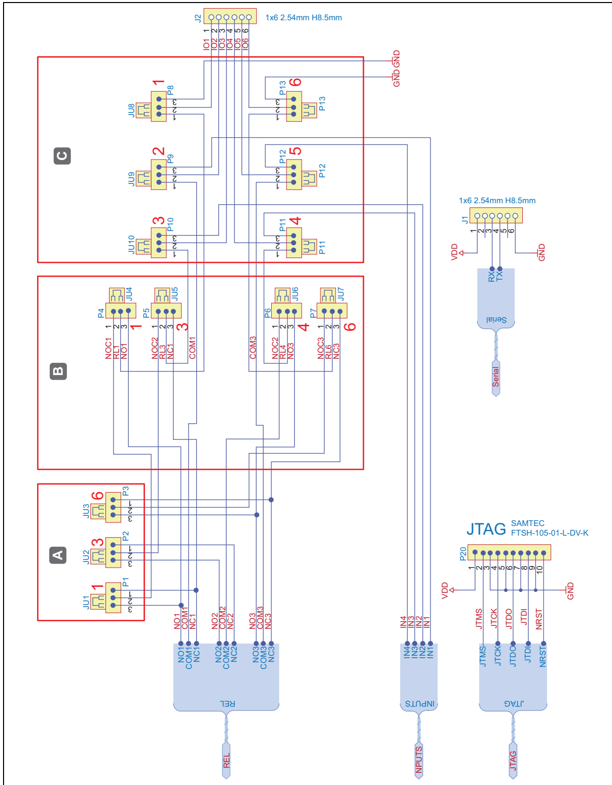
Ilustr. 16: Estructura y asignación de pin del WTX 200
