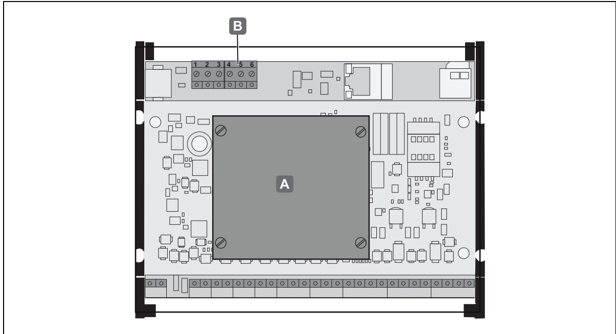
Fig. 15: Ligações com WTX 200
