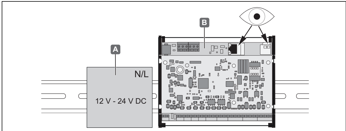
Fig. 5: Montaggio WTC 200
