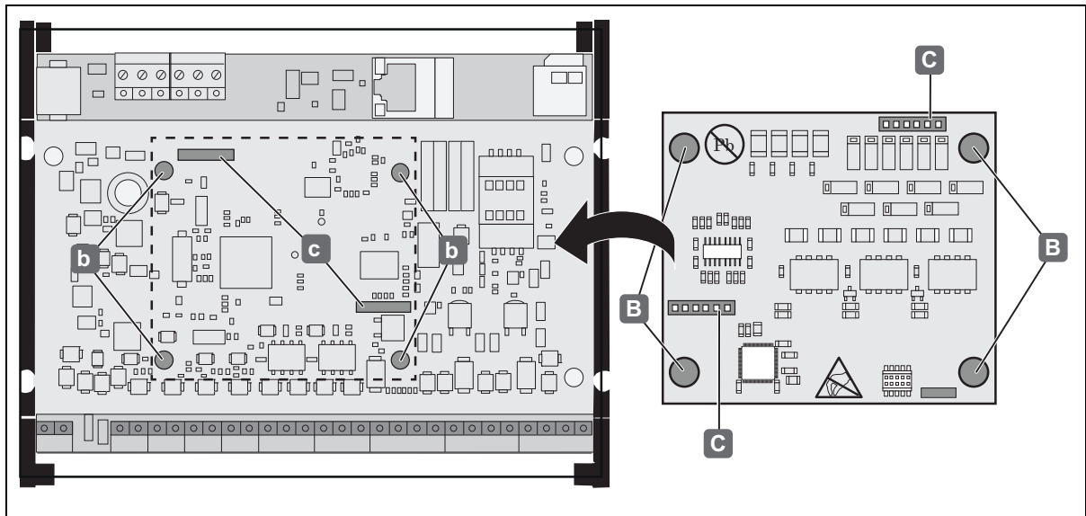
Abb. 9: Montage WTX 200 - WTX 200 auf Controller WTC 200 aufstecken
