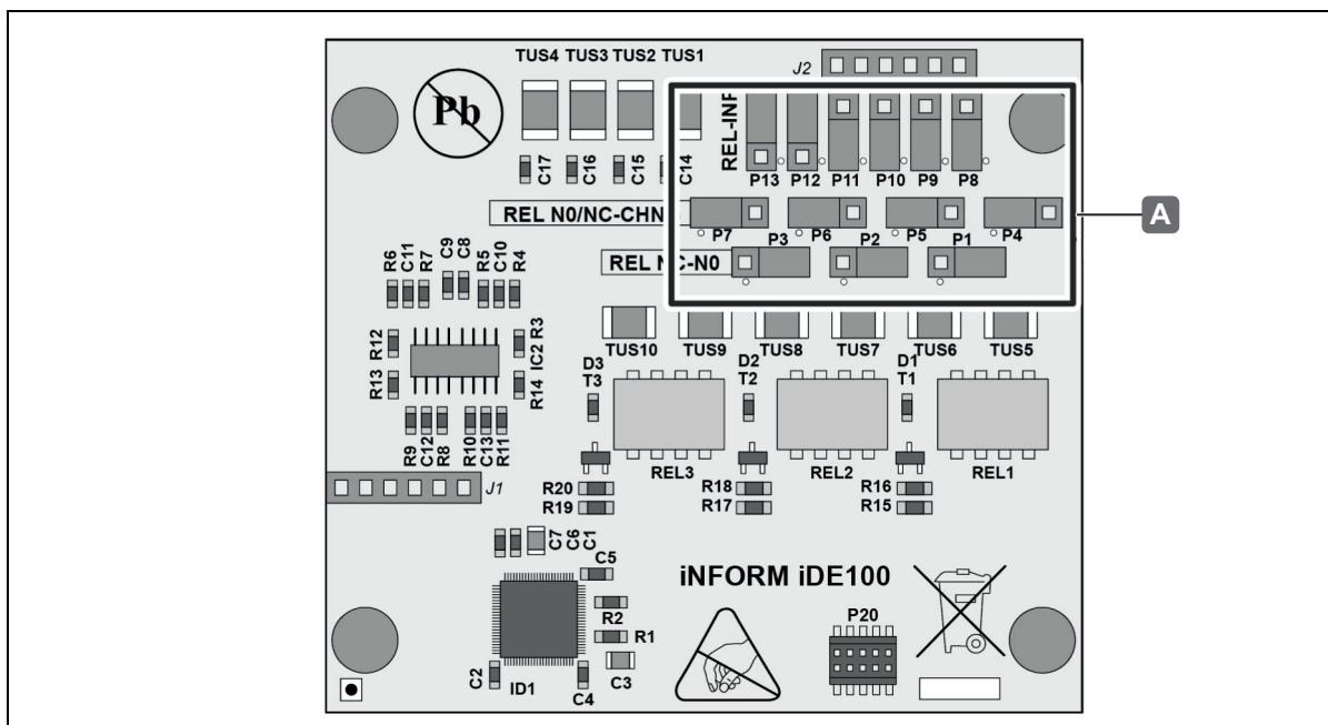
Fig. 19: WTX 200 - posição dos conectores quando utilizado para 2 portas de saída do relé adicionais e 1 porta de entrada analógica/digital adicional
