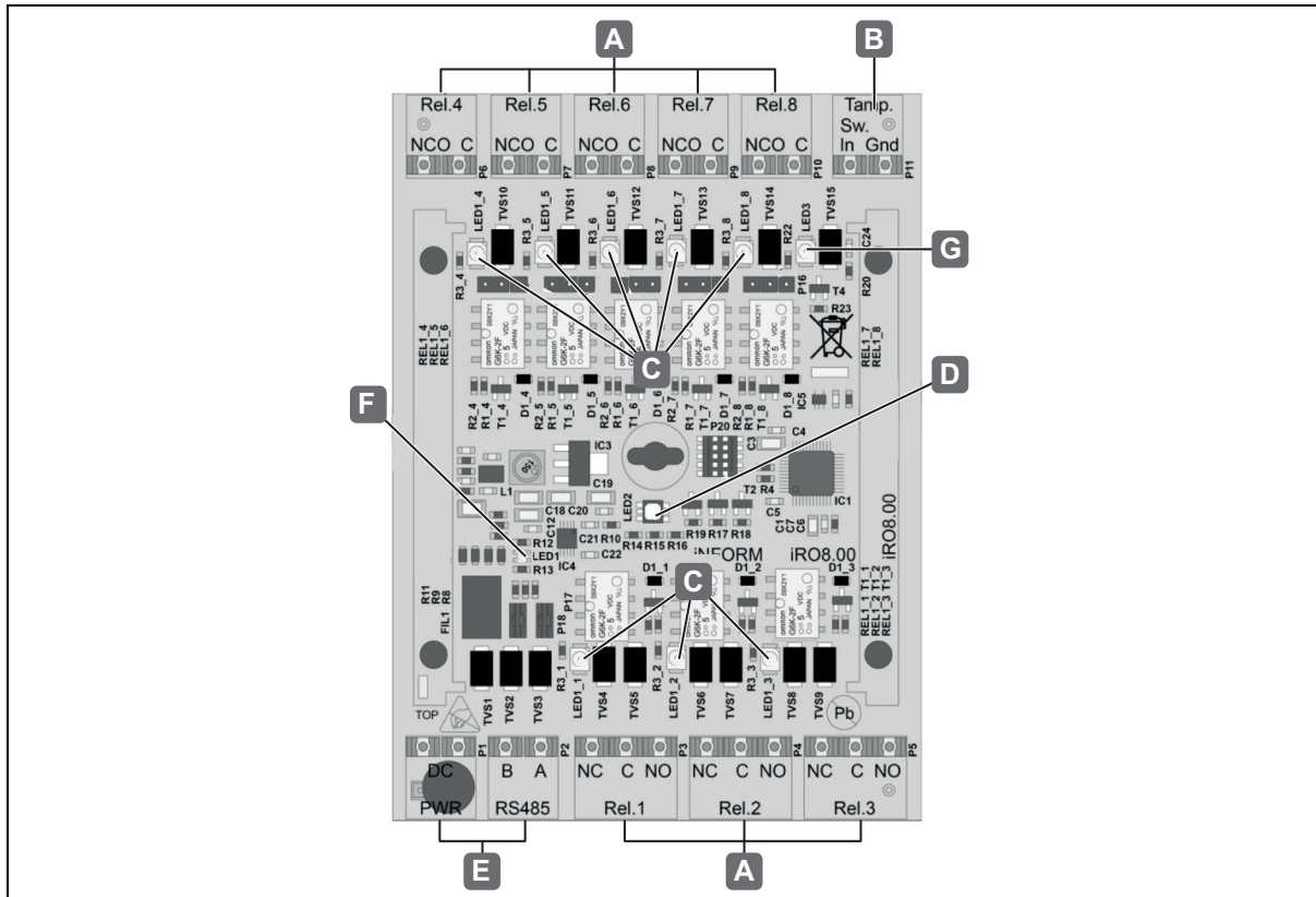
Fig. 20: Connexions WTX 201
