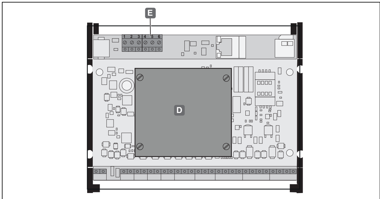
Ilustr. 10: Montaje WTX 200 - insertado en el controlador
