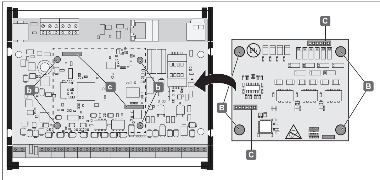
Fig. 9: Montaggio WTX 200 - WTX 200 inserire sul WTC 200 controller
