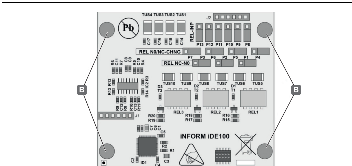
Ilustr. 8: Montaje WTX 200 - montar el distanciador
