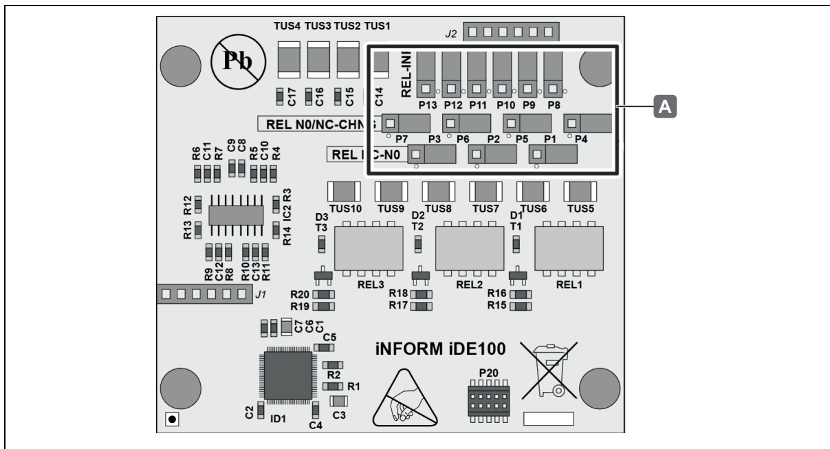
Fig. 18: WTX 200 - Position des cavaliers en cas d'utilisation pour des entrées analogiques/numériques supplémentaires
