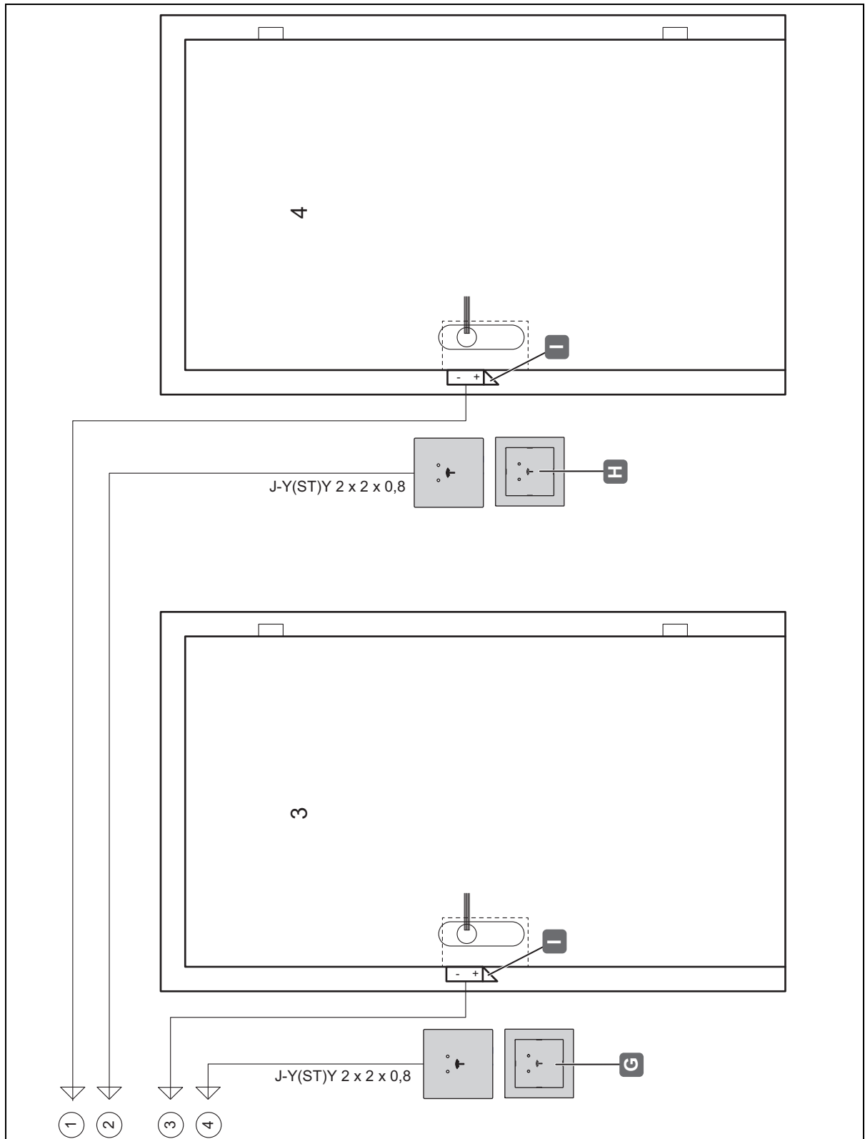
Abb. 32: Installationsbeispiel 5 - Teil 2 - Vier Türen mit je einem Leser / Türöffner und einem Controller (inkl. Erweiterungsboard)
