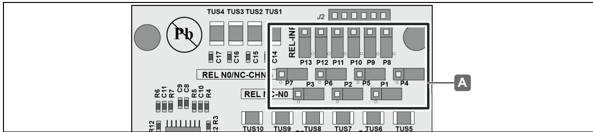
Ilustr. 7: Montaje WTX 200 - conectar los puentes
