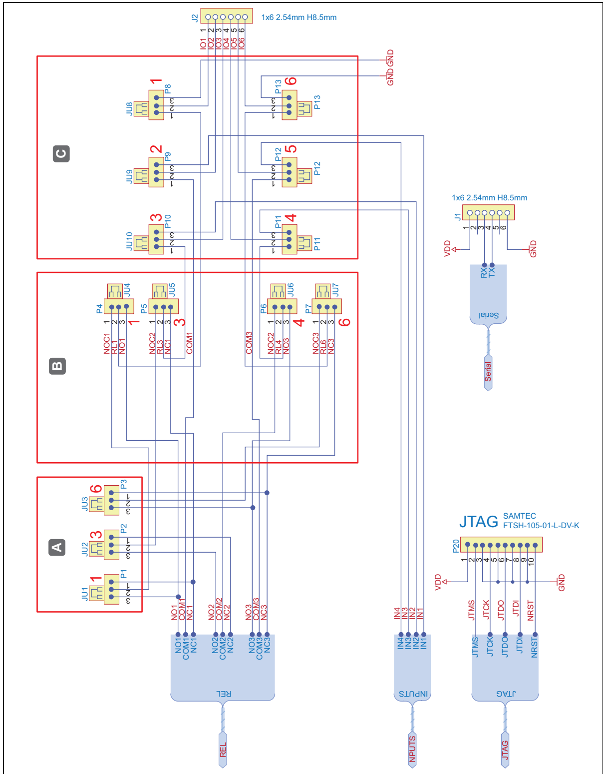
Abb. 16: Aufbau und Pin-Belegung des WTX 200
