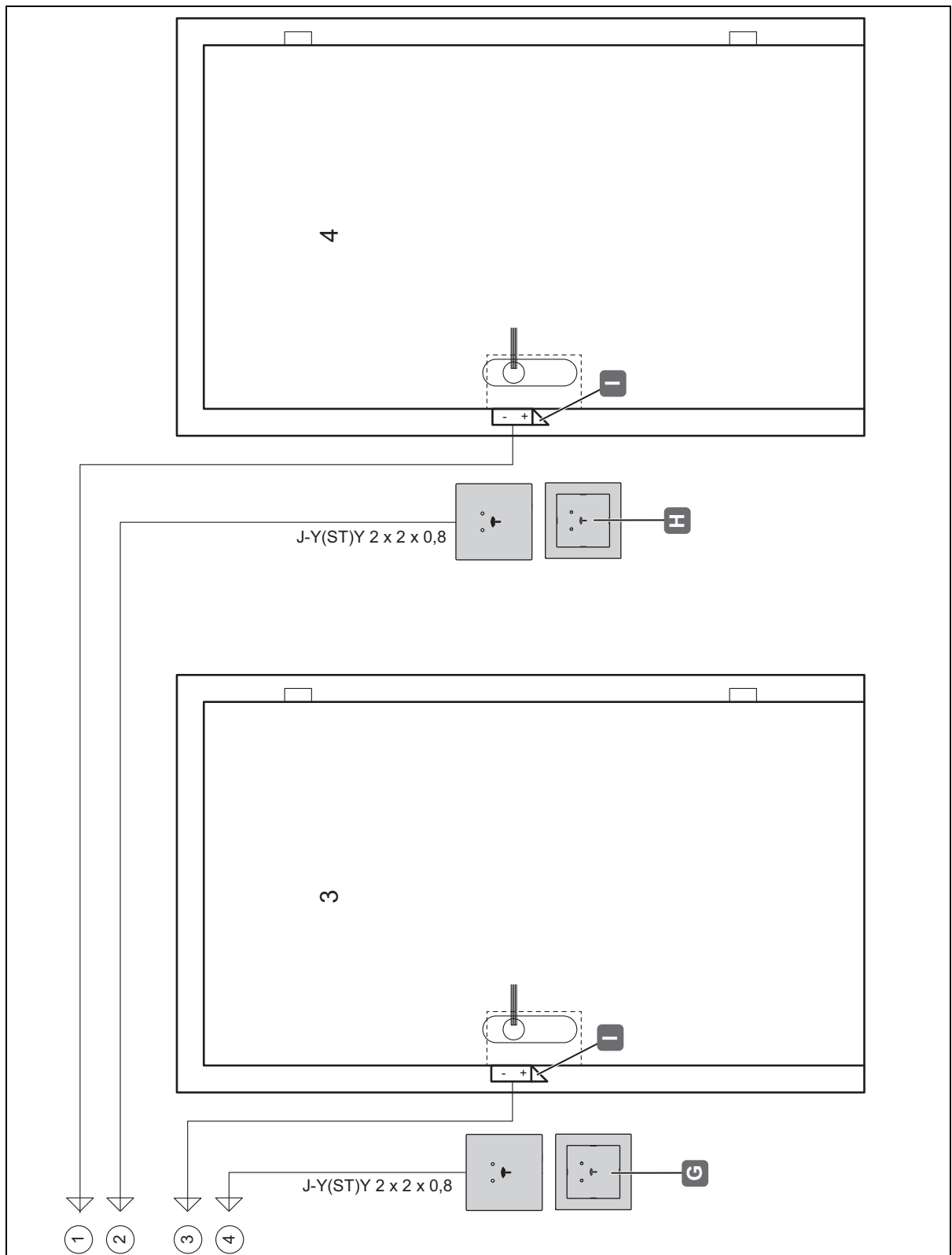
Fig. 32: Exemple d'installation 5 - Partie 2 - Quatre portes avec un lecteur/ouvre-porte chacune et un contrôleur (avec carte d'extension)
