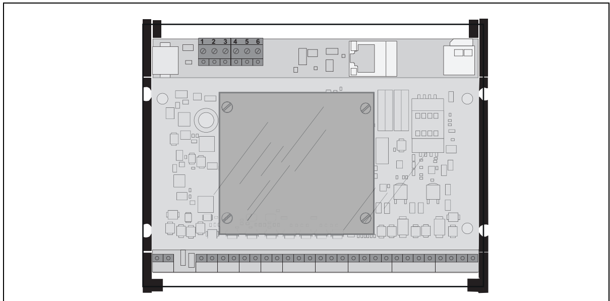
Ilustr. 3: WTX 200 - insertado en el controlador
