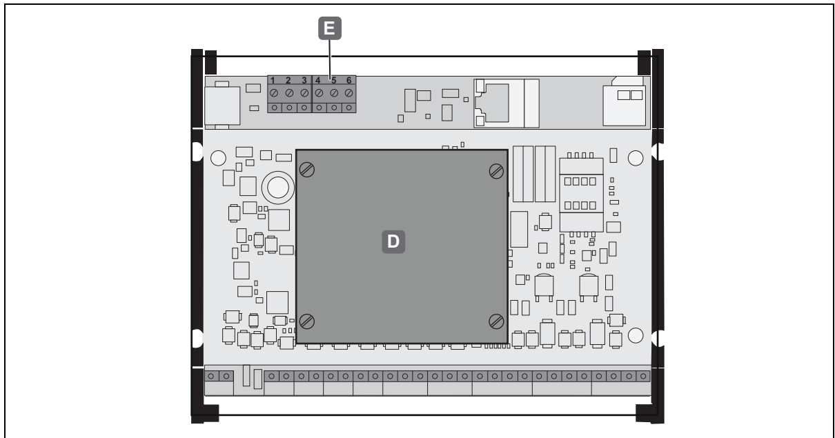
Fig. 10: Montage WTX 200 - enfiché sur le contrôleur
